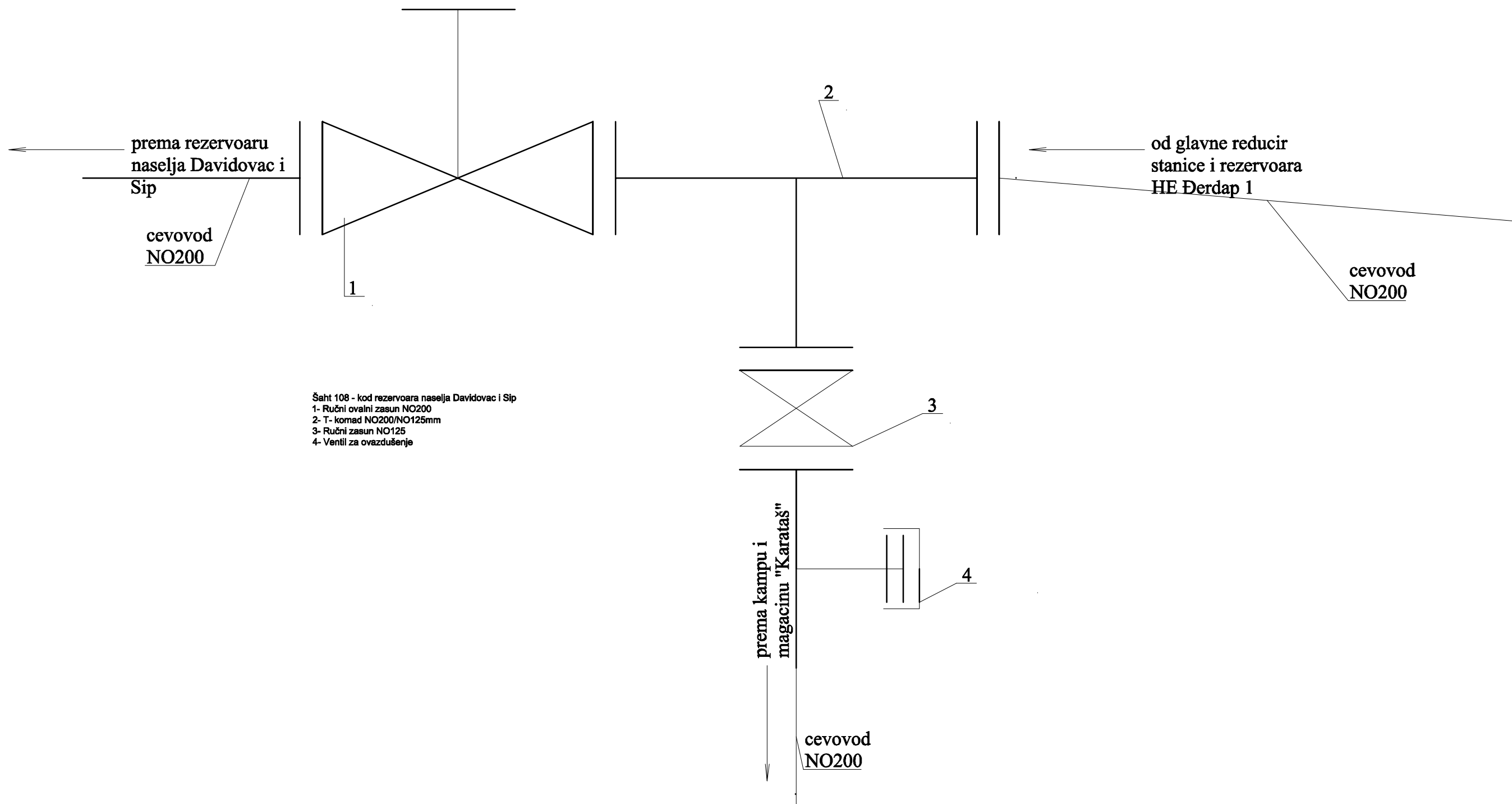
Crtež br.3 - Šaht na koti 108m - veza sistema za snabdevanje HE Đerdap 1 pitkom vodom sa dopunskim rezervoarom naselja Sip i Davidovac i kampu i magacinom
