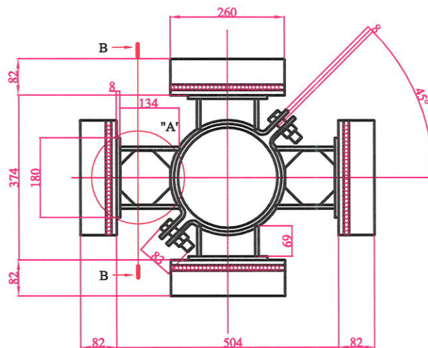
Vodeći oslonac VO-B
